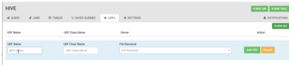
Figure 6.15. UDF Tab
